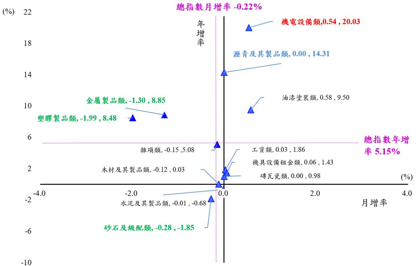
圖3、115年7月高雄市營造工程物價指數月增率及年增率
