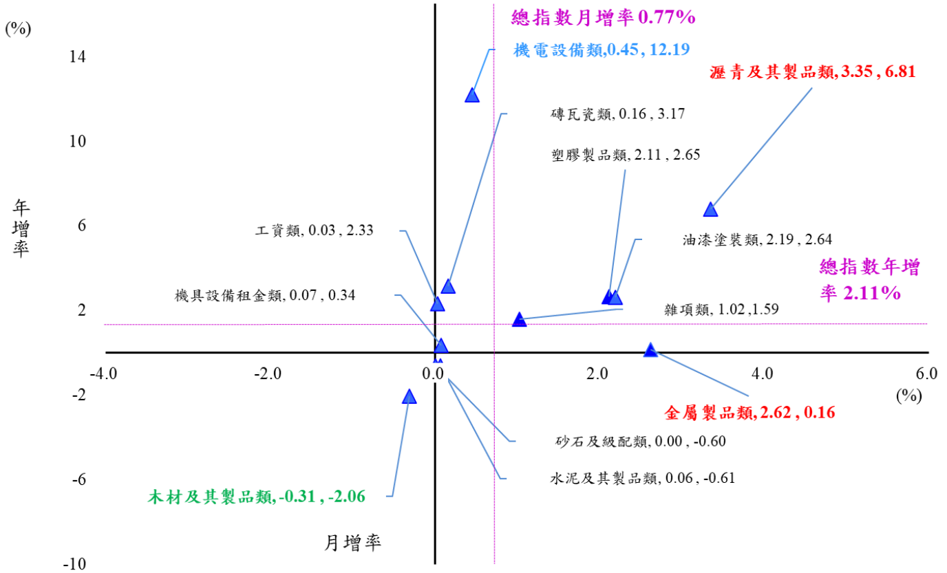
圖3、115年3月高雄市營造工程物價指數月增率及年增率
