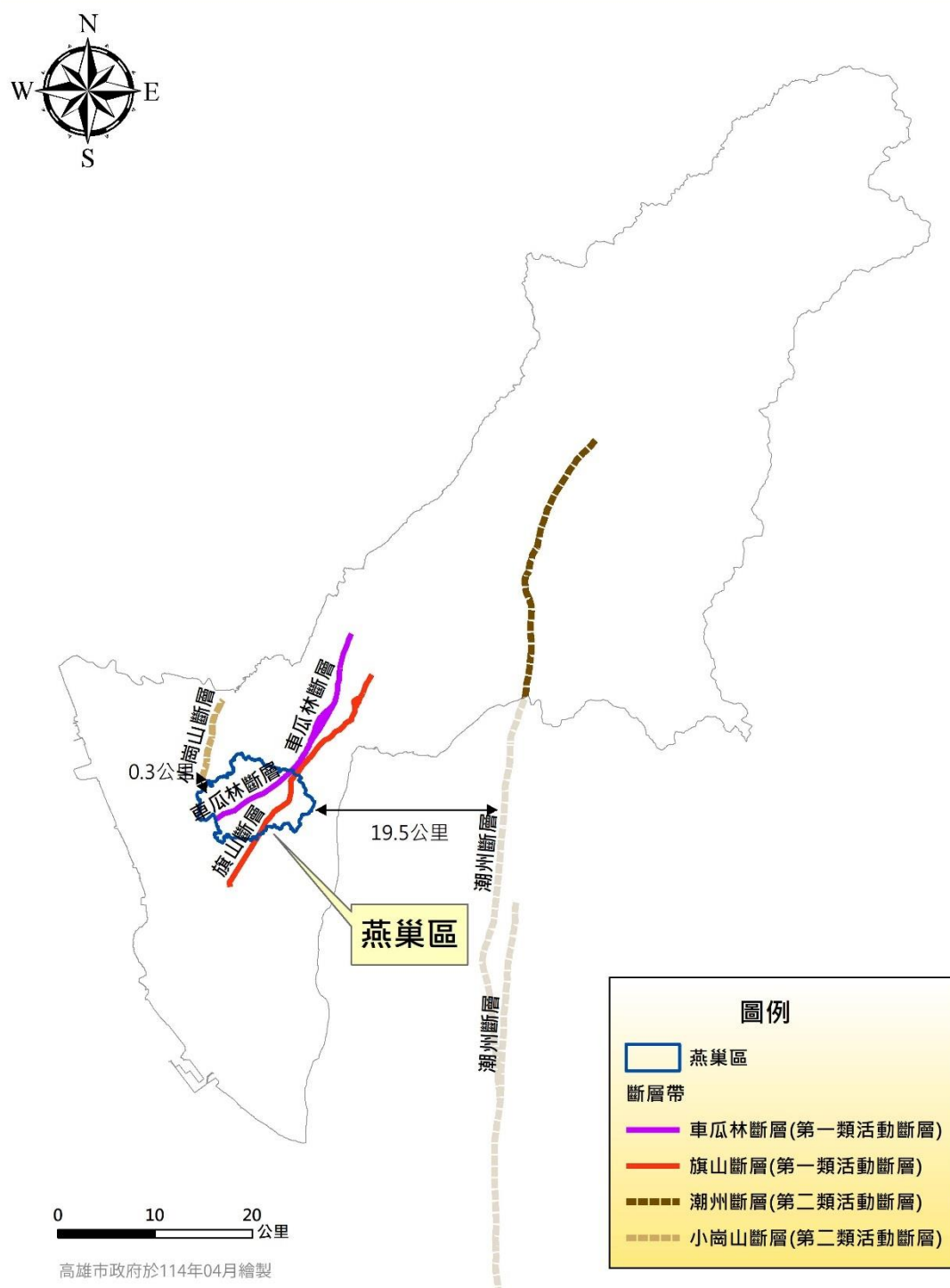
圖 14 燕巢區與高雄市斷層分布相對位置圖
