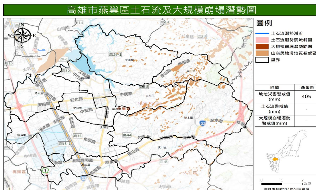
圖 12 燕巢區土石流及大規模崩塌災害潛勢圖
