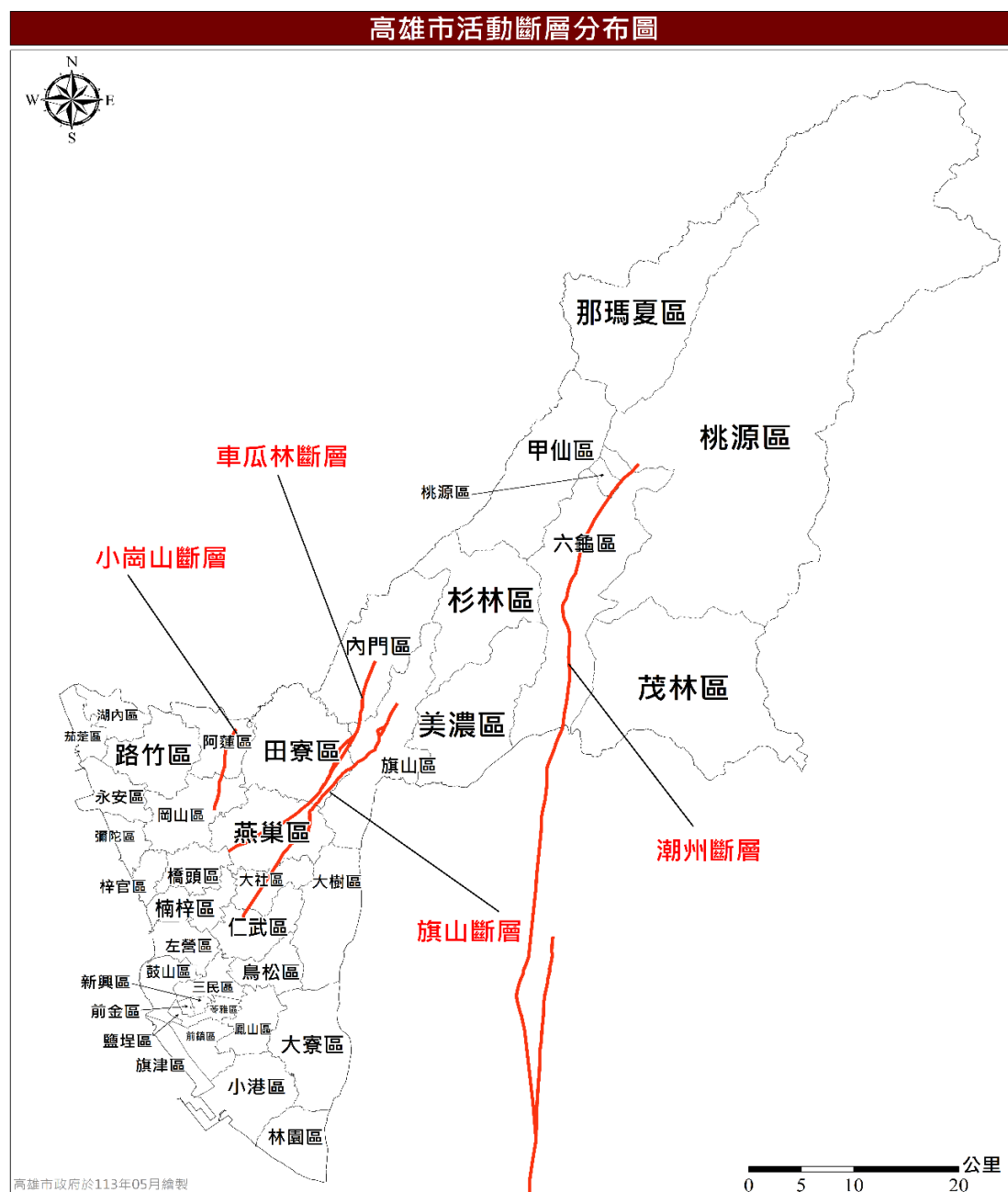
圖 13 高雄市境內與鄰近地區斷層分布圖
