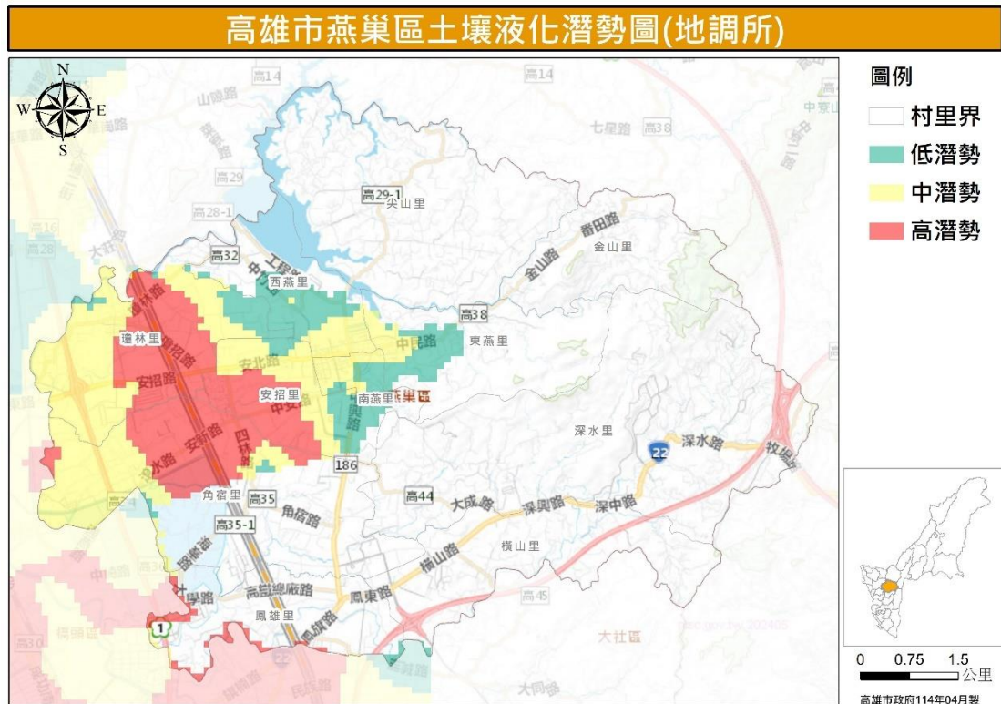
圖 27 燕巢區土壤液化潛勢圖（資料來源：地質調查及礦業管理中心）
