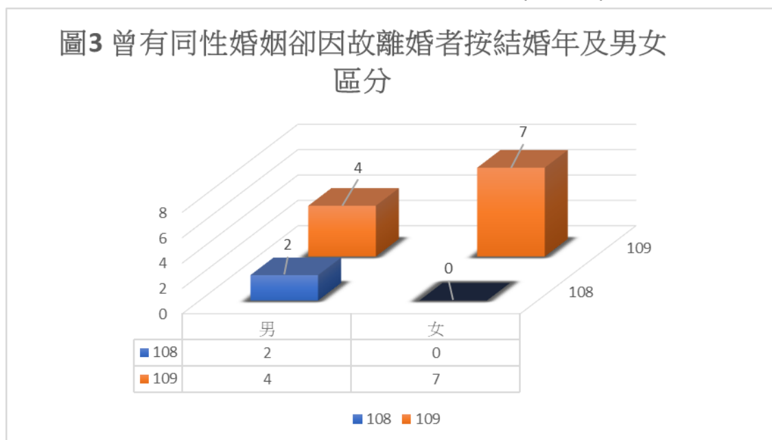
圖 3 曾有同性婚姻卻因故離婚者按結婚年及男女區分
