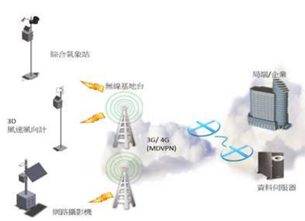
圖 3-40、文化資產保存環境監測設備通訊架構圖
