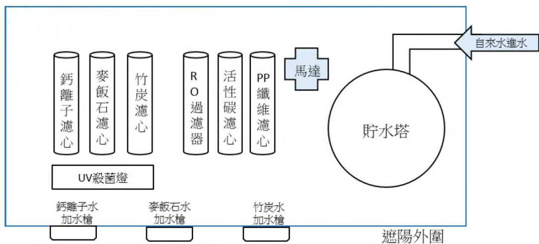
加水站設備配置圖
